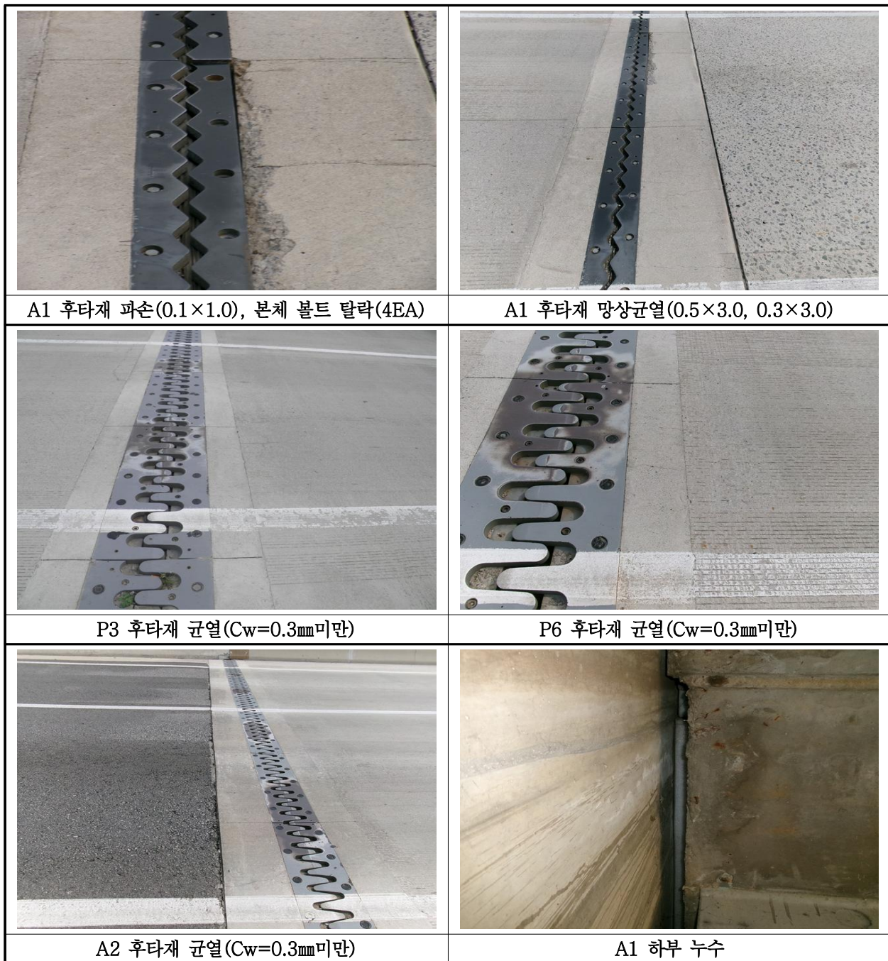
【사진 34.3.17】 신축이음장치 손상현황
