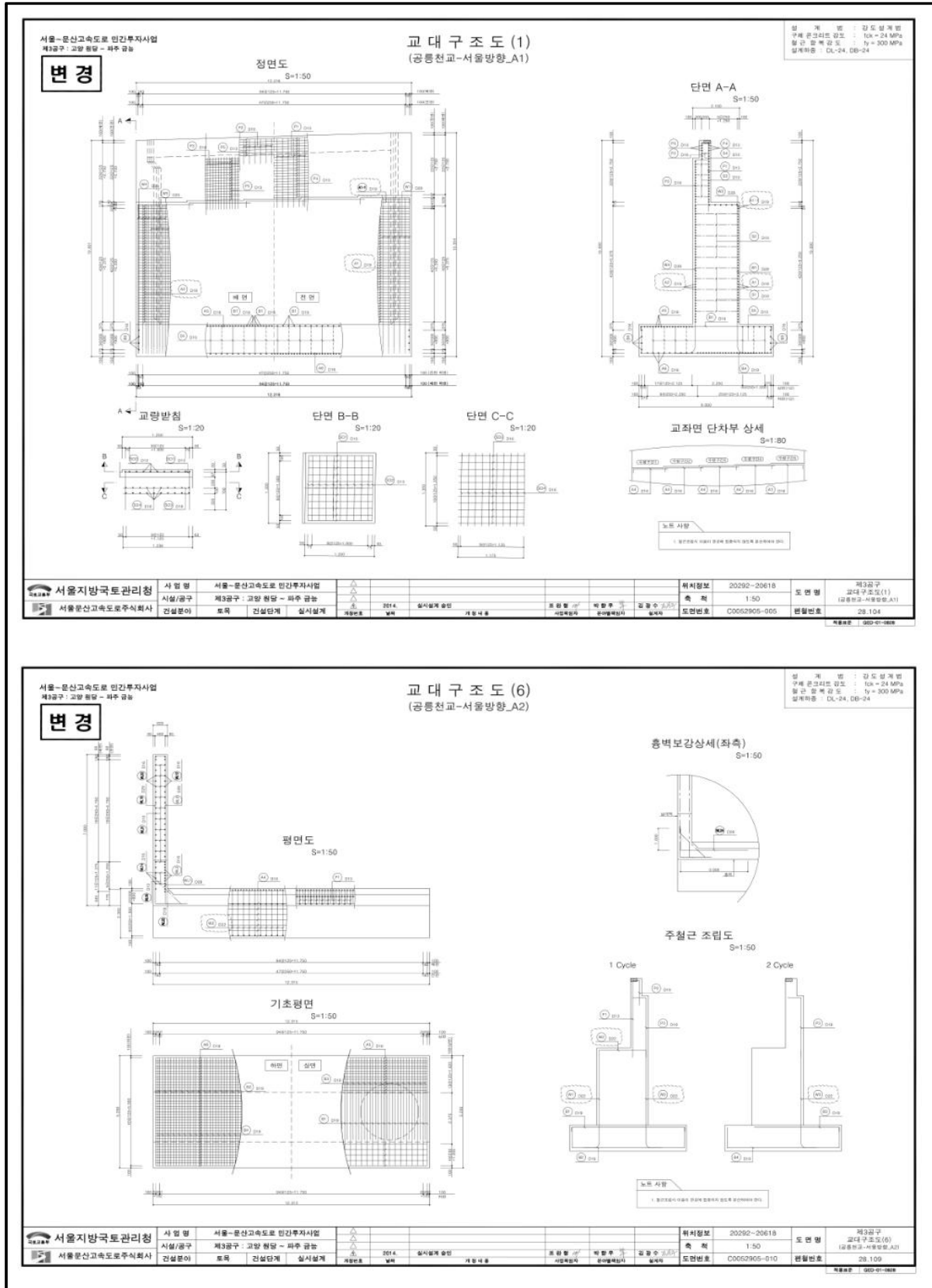
【그림 34.1.9】 교대 배근도
